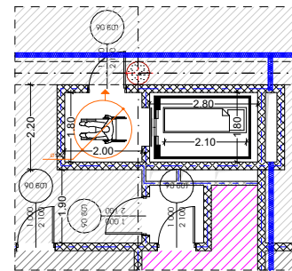
გეგმა -4.50 ნიშნულზე
