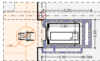
გეგმა 0.00 ნიშნულზე
