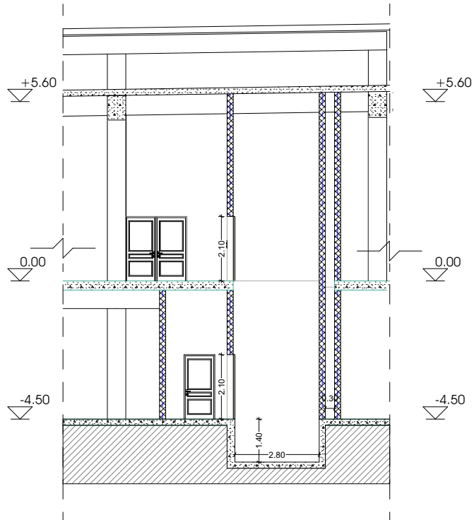
ჭრილი 3-3
